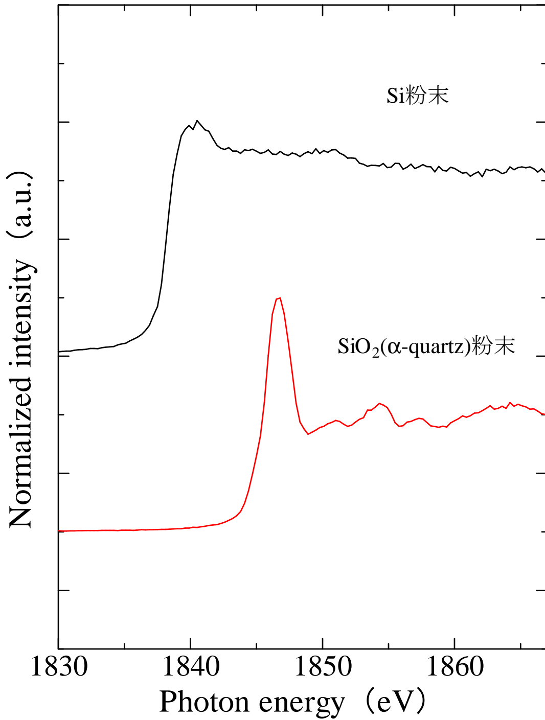
Si- K 吸収端XANESスペクトル（蛍光収量法）
