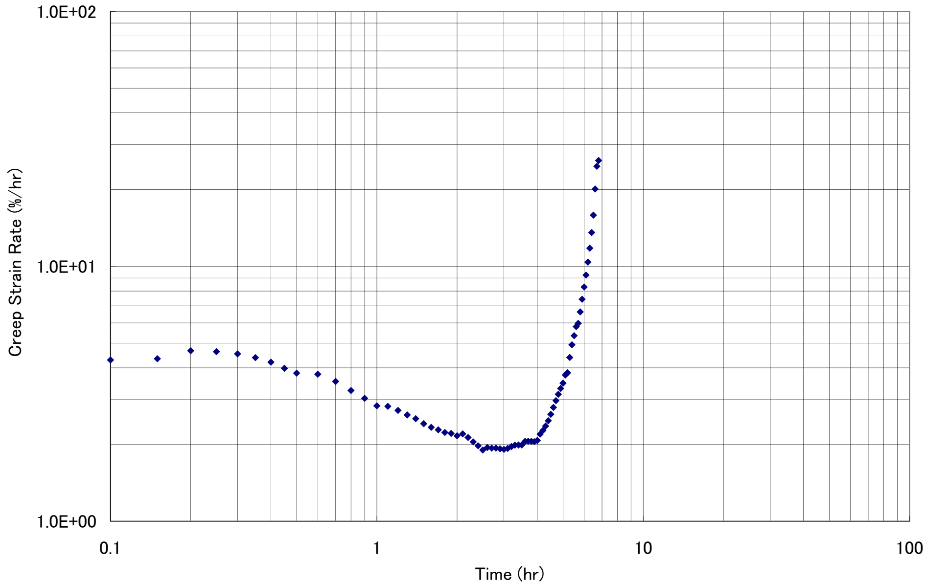
図 クリープ速度-時間曲線
